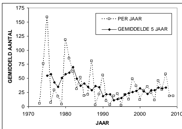
Figuur 5. Gemiddeld aantal Kauwen in de maanden januari en februari, zonder de Oosterveent
