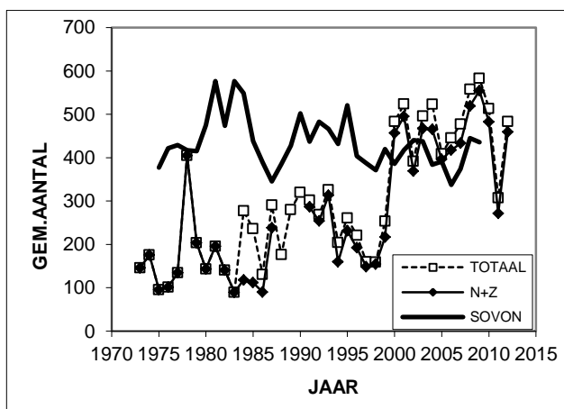
Figuur 3. Gemiddeld aantal getelde meerkoeten in februari t/m maart per jaar. De getrokken lijn geeft de aantallen zonder de Oostermeent, de stippellijn de totale aantallen en de dikke lijn de de aantallen van de watervogeltellingen van SOVON gedeeld door 200..
