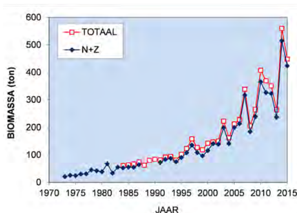
figuur 4 Het totaal van de waargenomen biomassa aan vogels met (totaal) en zonder de Oostermeent
