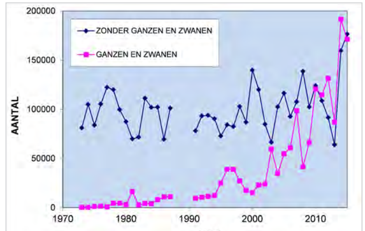
figuur 3 De getelde aantallen in de telgebieden Noord en Zuid van de ganzen en zwanen t.o.v. de andere soorten
