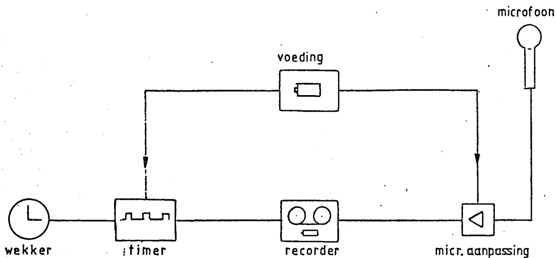
Figuur 1: Blokschema
